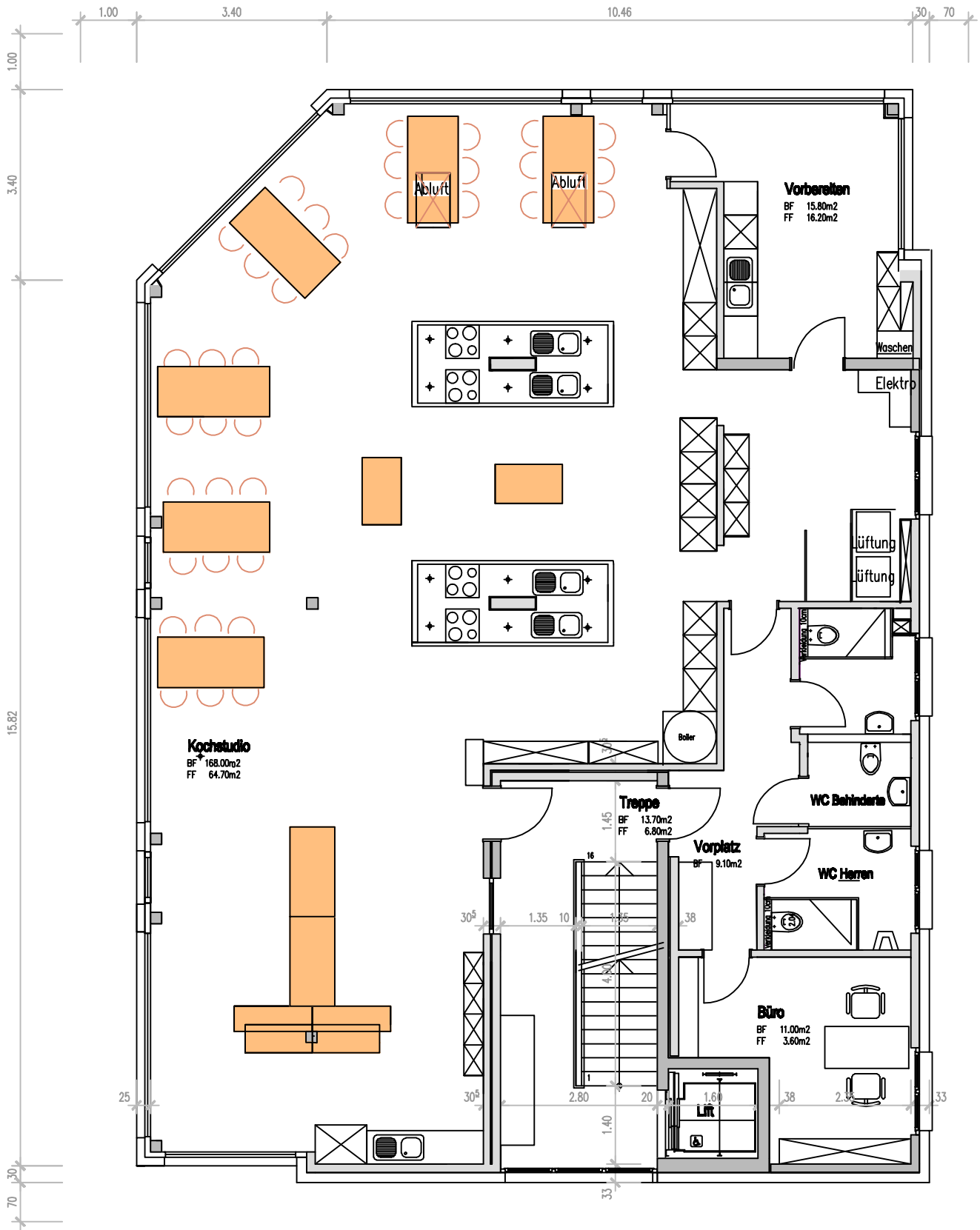
Grundriss Obergeschoss Mst. 1:100
